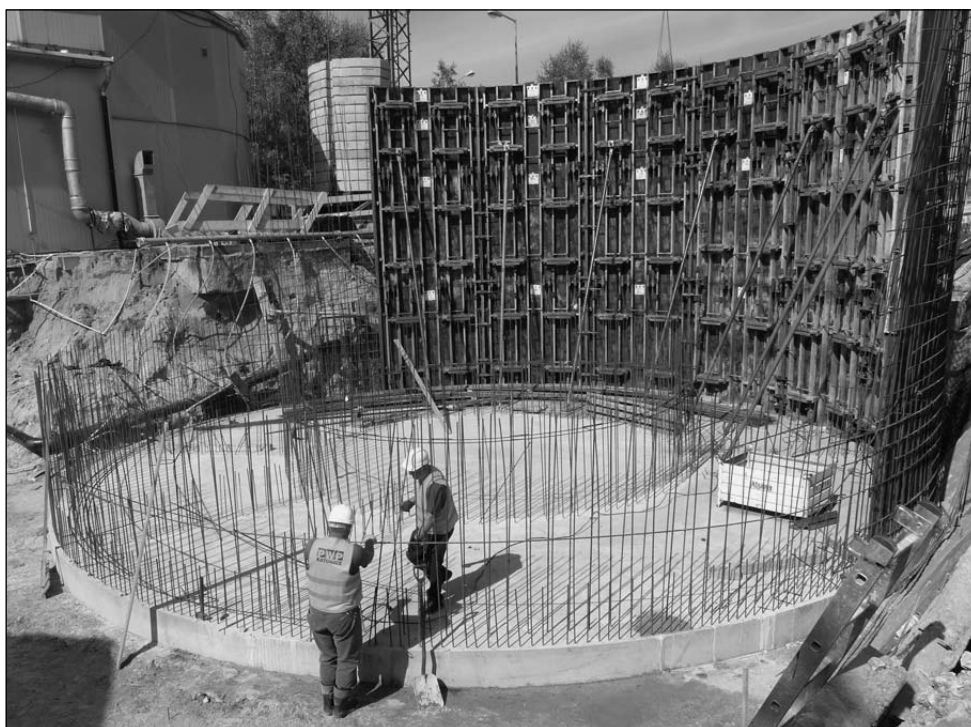
Przy ul. Wandy trwa budowa drugiego reaktora - bliźniaczego do istniejącego już w oczyszczalni ścieków.
